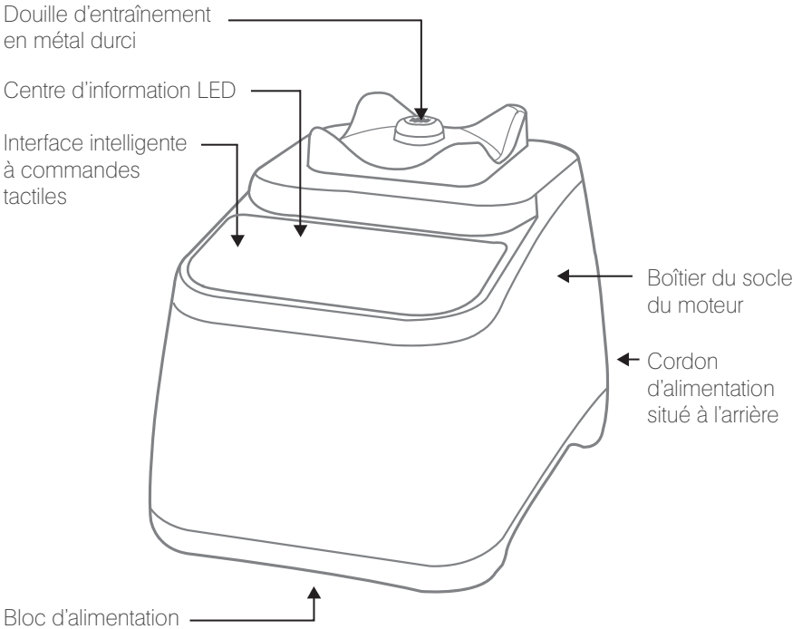
FIGURE 2: SOCLE DU MOTEUR
